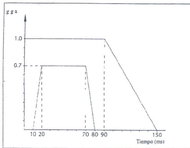
Figura - Envolvente cronológica de la aceleración
