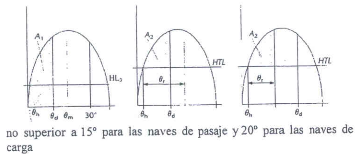
Figura 2 - Estabilidad con avería
